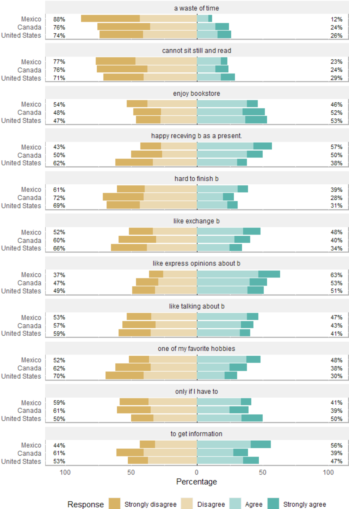
Fig. 4: Variabili di raggruppamento: grafico
